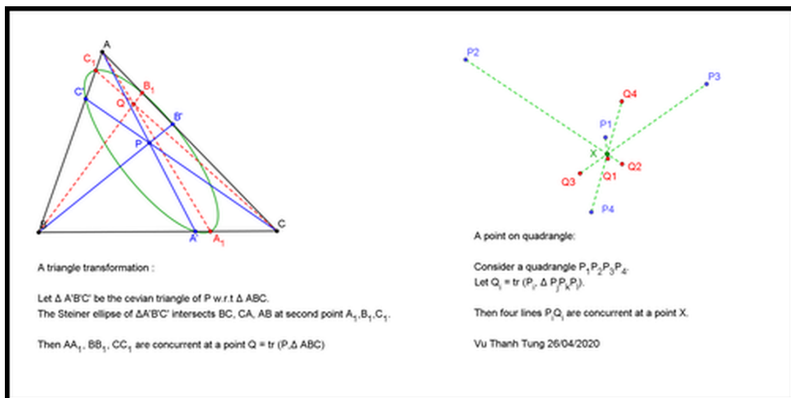
NewPointSteinerEllipse.png
